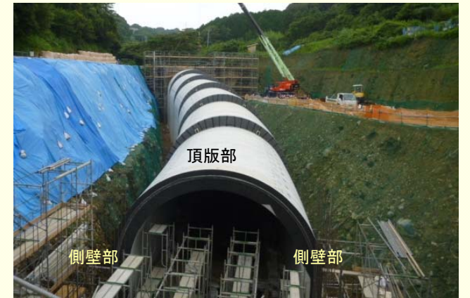
函渠工事施工状況(H27.7.2撮影)
