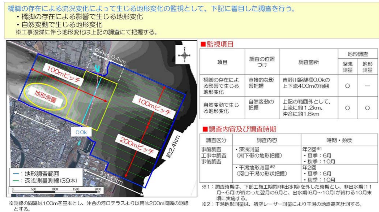
図 4.2-1 地形調査の調査計画
