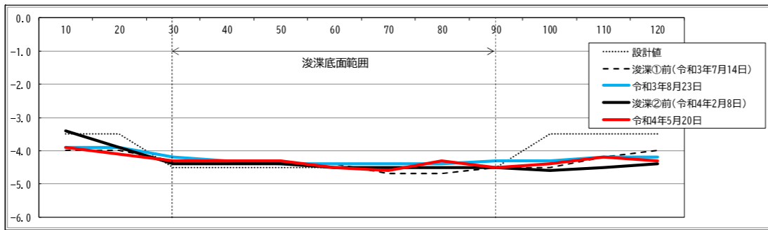
測線 A-A'
