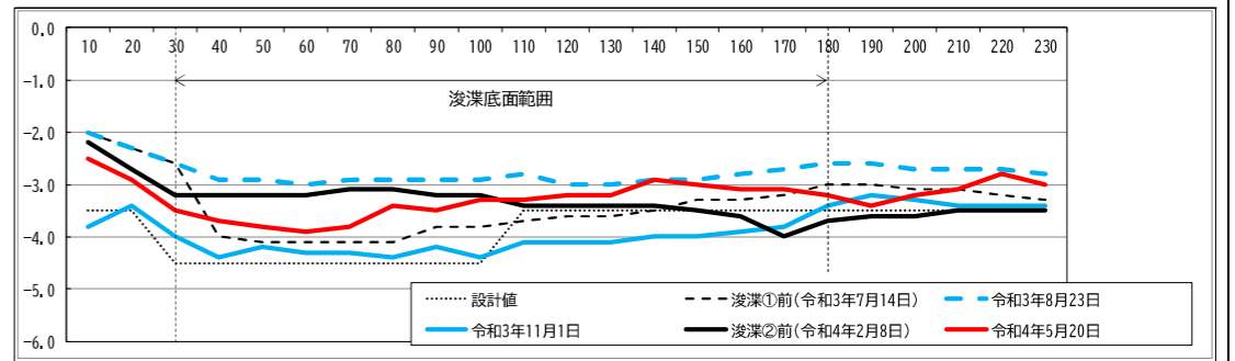
測線 B-B'
