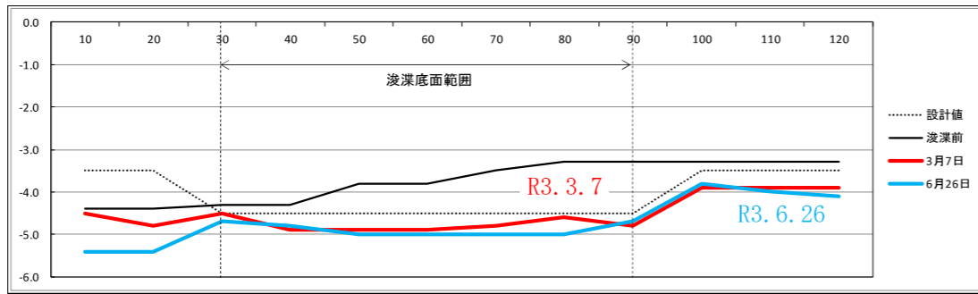
測線 C-C'
