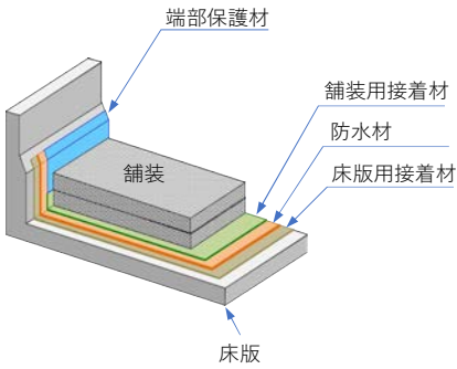
図 - 床版防水工断面図
