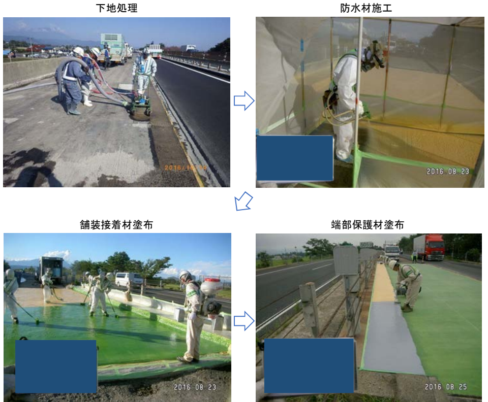
写真は、床版防水工（グレードⅡ）塗膜系防水の施工状況を示す。
