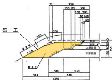
図 - 舗装端部
